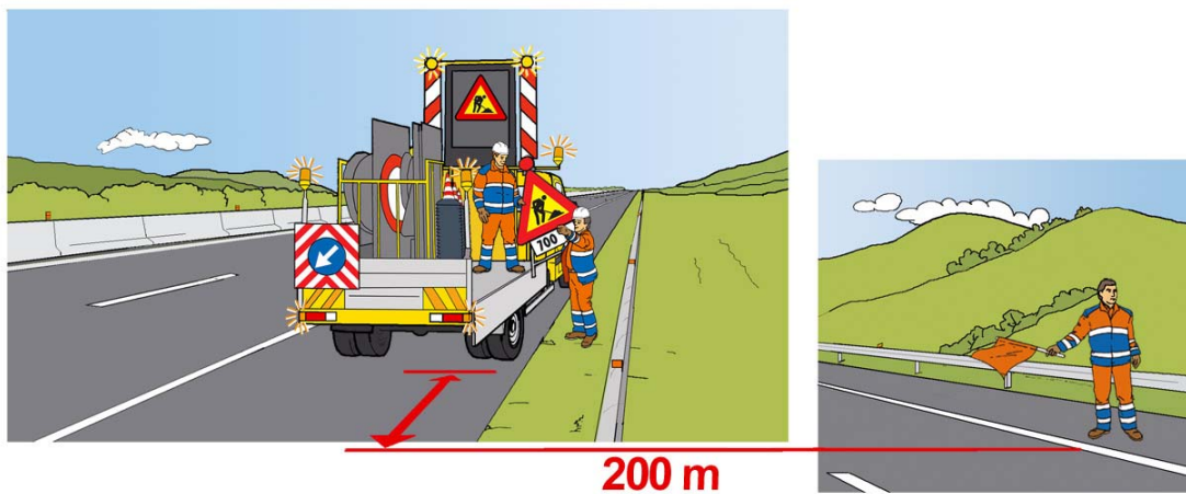
Figura 27 – Chiusura della corsia di marcia: scarico ed installazione del segnale lavori sul margine destro
