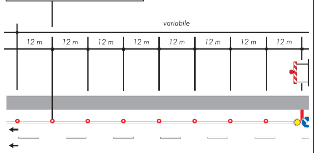
fig. 8 Segnaletica di posizione – delimitazione longitudinale dell'area interessata dal cantiere realizzata con coni o delineatori flessibili
